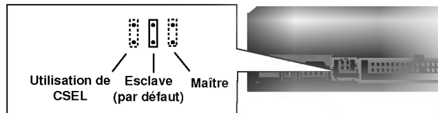
Figura 3.Cavalier de configuration de l'unité
