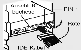
Abbildung 9. Verbinden des IDE Kabels mit der Schnittstelle
