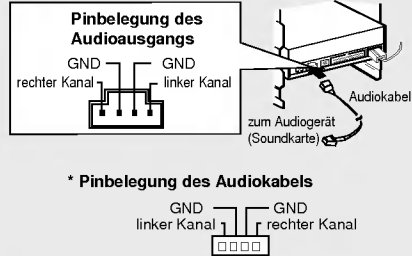
Abbildung 10. Verbinden des Audiokabel mit der Audioausgangsbuchse
