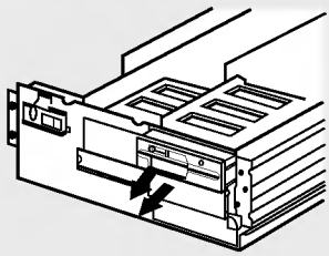
Figura 6. Desmontando la disquetera y las chapas de sujeción
