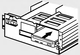
Figura 7. Montando la unidad
