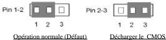
Figure 2-8. Paramètre du CCMOS1
