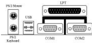
Figure 2-10. Connecteurs d’entrées/sorties de votre ZM6.
