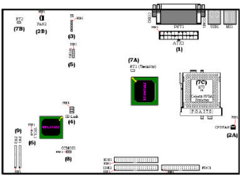
Figure 2-7. Dispositions de tous les connecteurs et broches sur la ZM6
