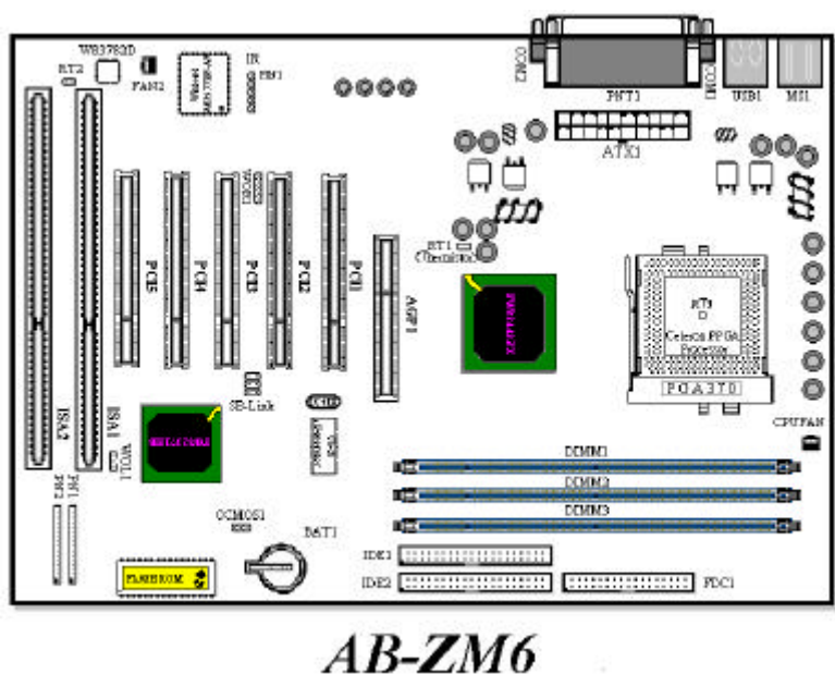
Figure 1-2 Emplacement des composants de la carte mère
