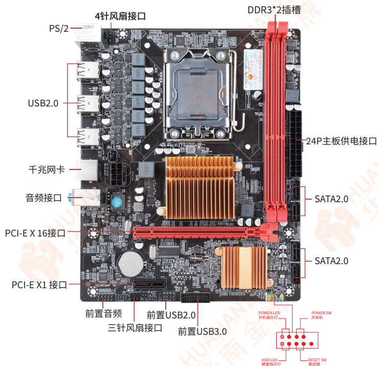
图1-1 X58-RX 2.0主板图解
