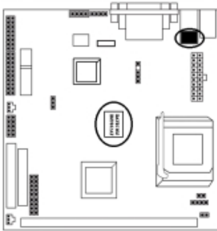
LAN Connector
