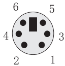
PS/2键盘接口
