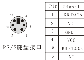
PS/2键盘接口针脚定义
