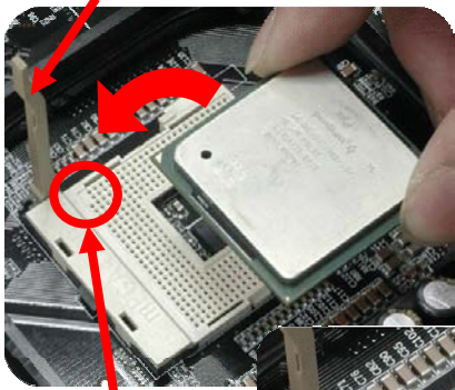
插座第一接腳
