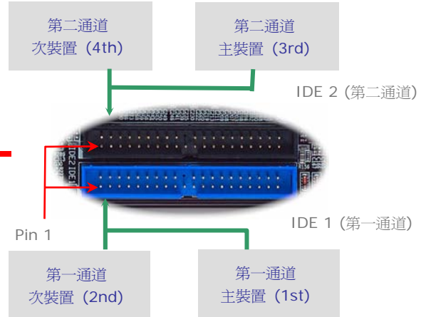
ATA 66/100/133 IDE 排線接頭
