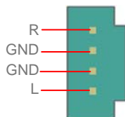
AUX-IN 接頭
