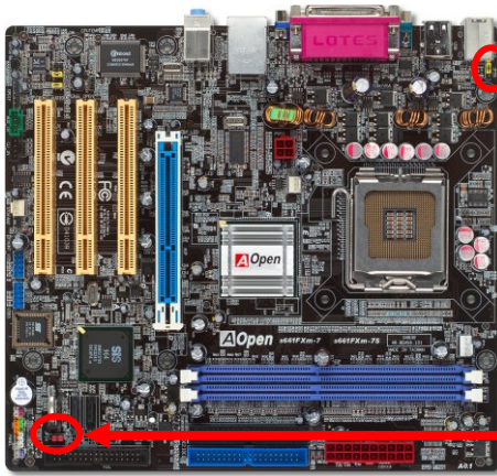
JP14 CMOS 清除跳線
