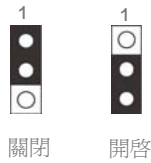
JP28 鍵盤/滑鼠喚醒功能跳線
