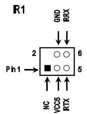
IR infrared module Headers
