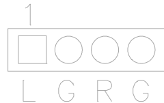
Fig. 10 CD-ROM Audio
