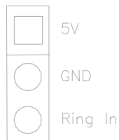
Fig. 11 Wake up On LAN
