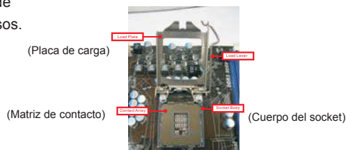
Introducción al socket de 1156 agujas
