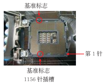
1156 针插槽
