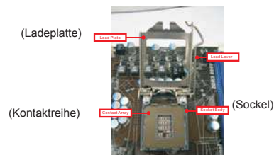
1156-Pin Sockel Übersicht
