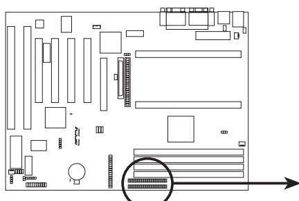
IDE Connectors
