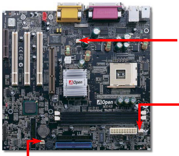
FAN3 コネクタ
