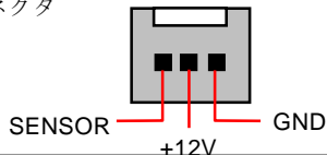
FAN3 コネクタ
