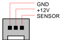
CPU ファンコネクタ
