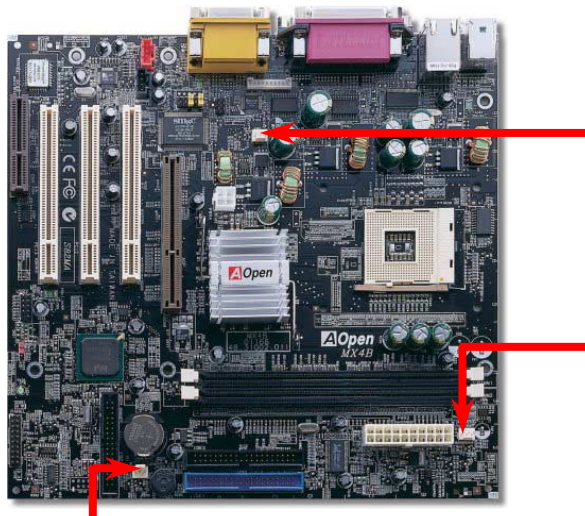
FAN3-Anschluss
