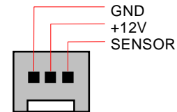
CPU Fan Connector
