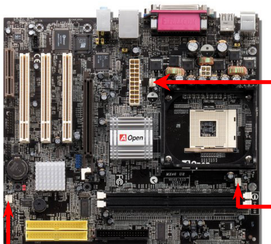
CPUFAN1 接頭
