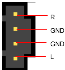
CD 入カコネクタ
