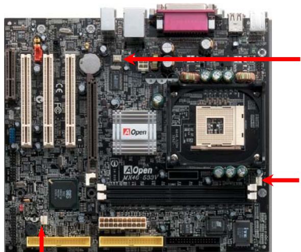
CPU FAN コネクタ
