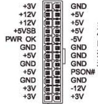
主供电接头
