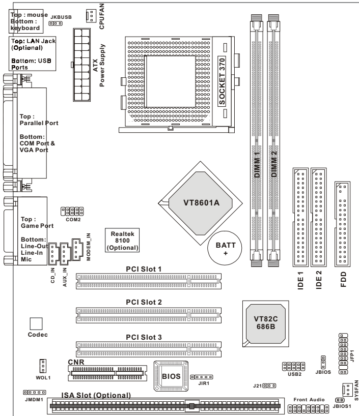
MS-6368 (v2.X) Micro-ATX VA Mainboard
