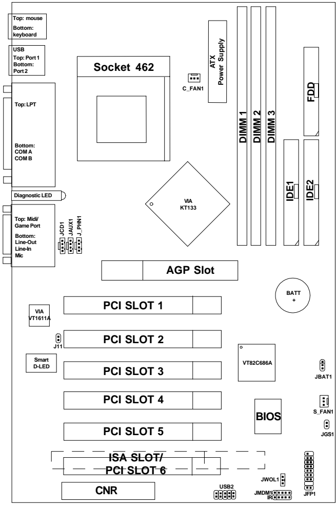
K7T Pro 2 (MS-6330) ATX VA Mainboard
