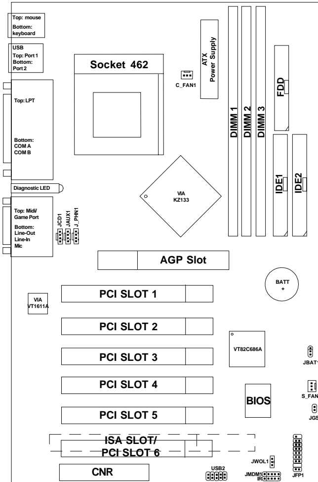
K7Z PRO(MS-6330) ATX VA Mainboard
