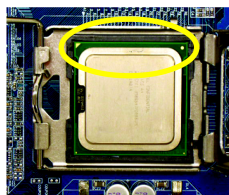
図 3 CPU ソケット端に位置する小さな金色の三角形に注目します。CPU の刻み目のある角を三角形に合わせ、CPU を静かに装着します。(CPU を親指と 4 本の指でしっかりとつかみ、直線的な下方動作でソケットに押し込みます。装着時に CPU の損傷を引き起こす可能性のあるひねりや曲げ動作は避けてください。)
