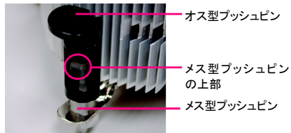
図2 (プッシュピンを矢印方向に向けると、CPUクーラーを取り外し、反対の方向は取り付けになります。)取り付け前に、オス型プッシュピンの矢印が内側を向かないように注意します。(この手順はIntel 梱包ファン向けのみ適用です)
