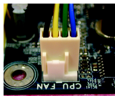
図6 最後にCPUクーラーの電源コネクタをマザーボードにあるCPUファンヘッダに接続します。
