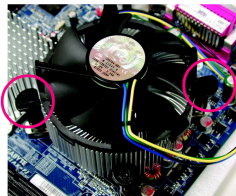
Abb. 3 Legen Sie den Kühlkörper oben auf die CPU und stellen Sie sicher, daß die Steckerstifte am Stiftloch des Motherboard ausgerichtet sind. Danach die Steckerstifte diagonal niederdrücken.
