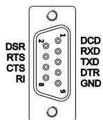
DB9针式插座引脚定义
