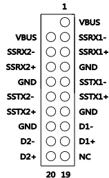
USB3.0 扩展式插针定义
