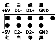
USB2.0 扩展式插针定义
