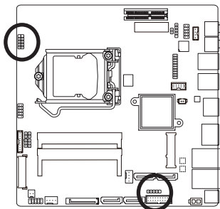
FUSB2_2/FUSB2_4
