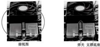
俯视图
