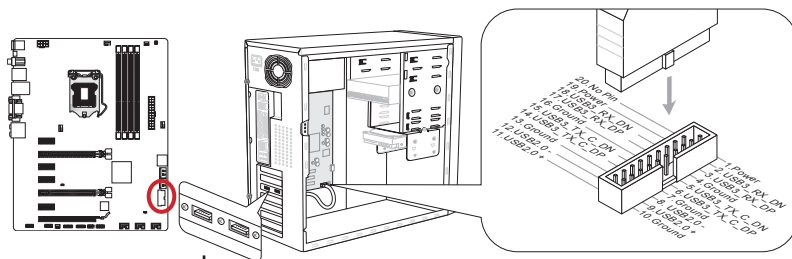
Выносная планка USB 3.0 (опционально)
