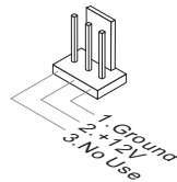
SYSFAN3/ SYSFAN4
