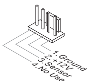
SYSFAN1/ SYSFAN2
