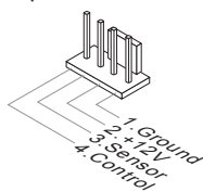
CPUFAN
