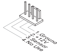
SYSFAN1/ SYSFAN2
