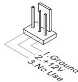
SYSFAN3/ SYSFAN4
