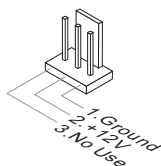
SYSFAN3/ SYSFAN4
