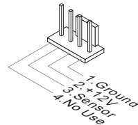
SYSFAN1/ SYSFAN2
