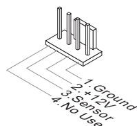
SYSFAN1/ SYSFAN2
