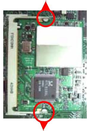
MINIPCI
