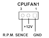
Fan Connector
