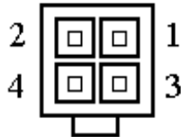
ATX_12V
