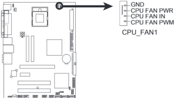
IMISR-VM CPU FAN CONNECTOR
