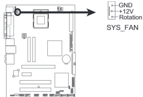
IMISR-VM SYSTEM FAN CONNECTOR
