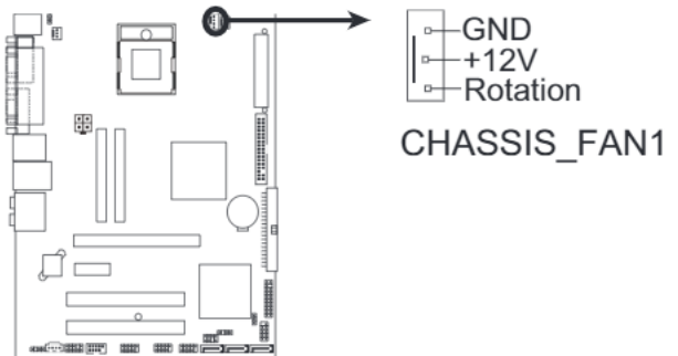
IMISR-VM CHASSIS FAN CONNECTOR
