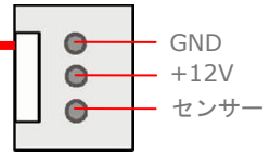
POWER FAN コネクター
