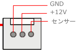
System FAN コネクター
