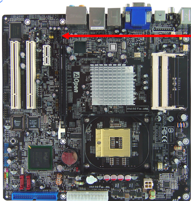
CD-INコネクタ
