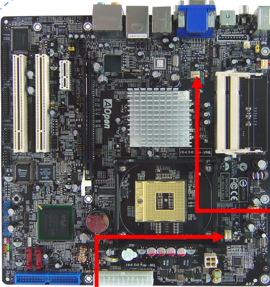
System FAN コネクター
