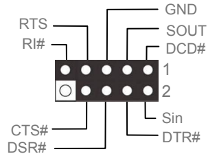
COM1コネクタ (i945Ga-PHSのみ)
