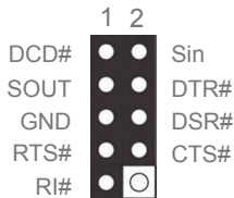
COM2コネクタ
