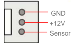
SYSFAN1 接頭
