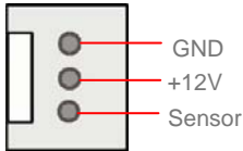
SYSFAN2 接頭
