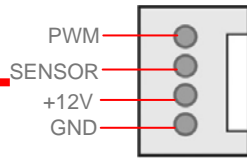
CPUFAN 接頭
