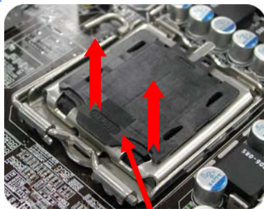
塑膠蓋
