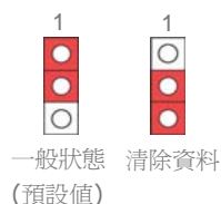
JP14 CMOS 清除跳線
