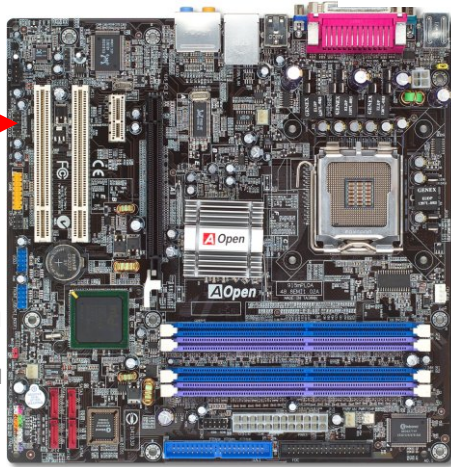
Front Audio 前音效接頭
