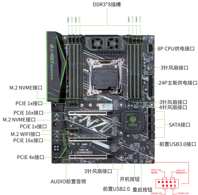
图1-1 X99-T8主板图解
