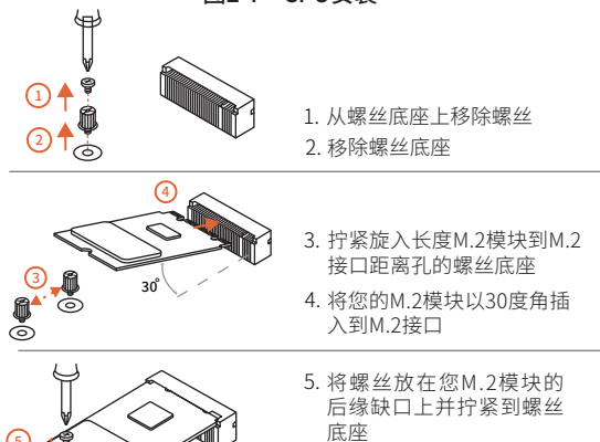
图2-7 CPU安装
