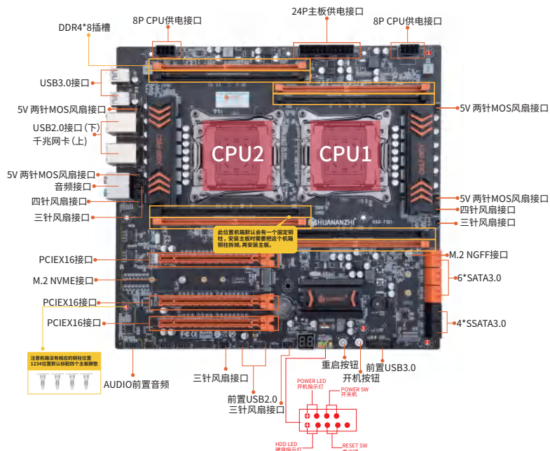
图1-1 X99-F8D主板图解
