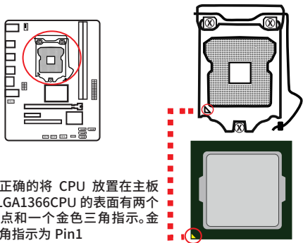
图2-6 CPU安装
