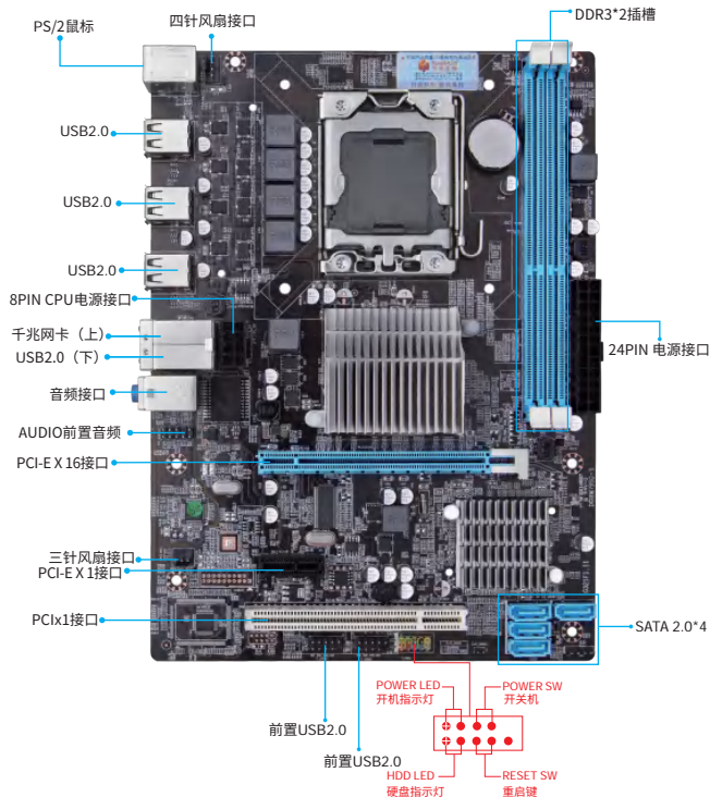
图1-1 X58 2.0主板图解
