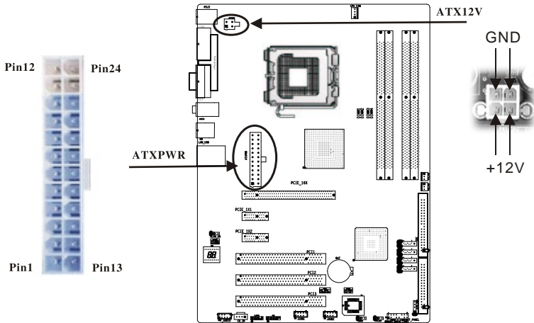
ATXPWR针脚定义
