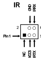
IR IR infrared module Headers
