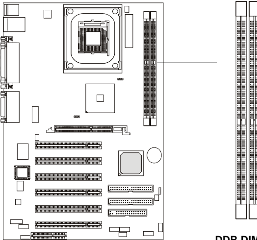
DDR DIMM Slots (DDR 1~2)
