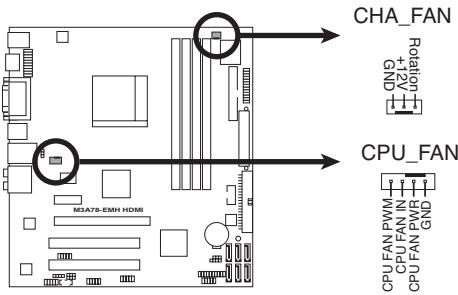
M3A78-EMH HDMI Fan Connectors
