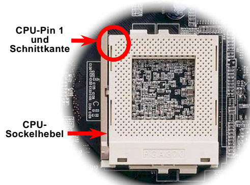
CPU-Schnittkante
