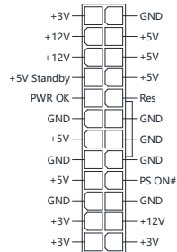
ATX_PWR
