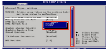
设置窗口
