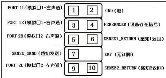
HD Audio 前置音频连接引脚定义
