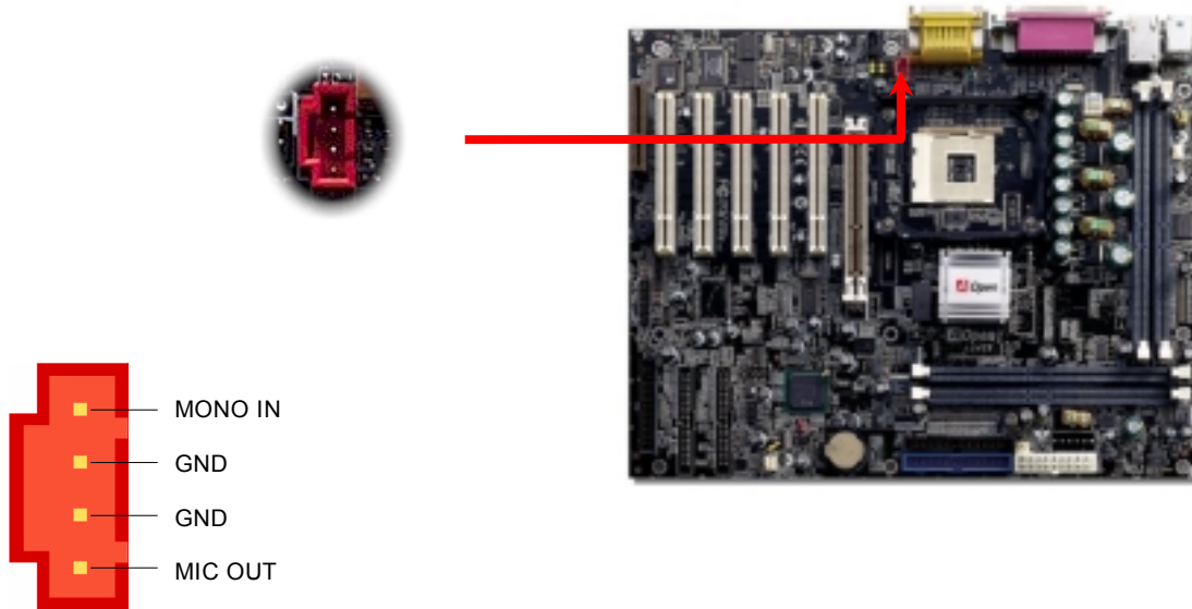
MODEM-CN-Anschluss
