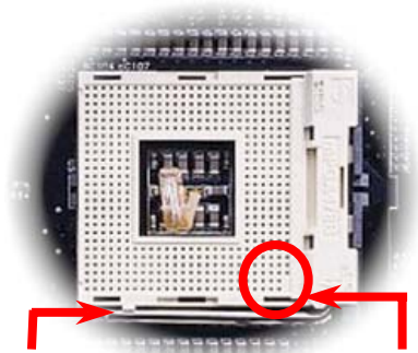
CPU 第一針腳位置
