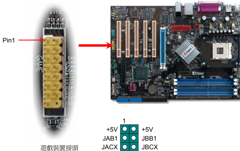
遊戲裝置接頭
