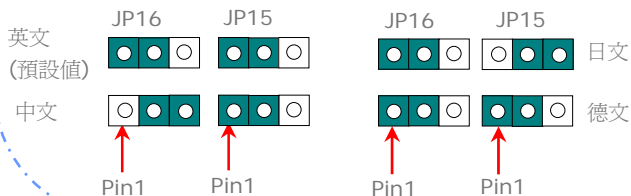
JP15/16 Dr. Voice 語言選擇跳線
