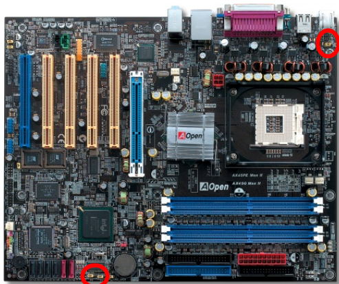
JP15/16 Dr. Voice 語言選擇跳線
